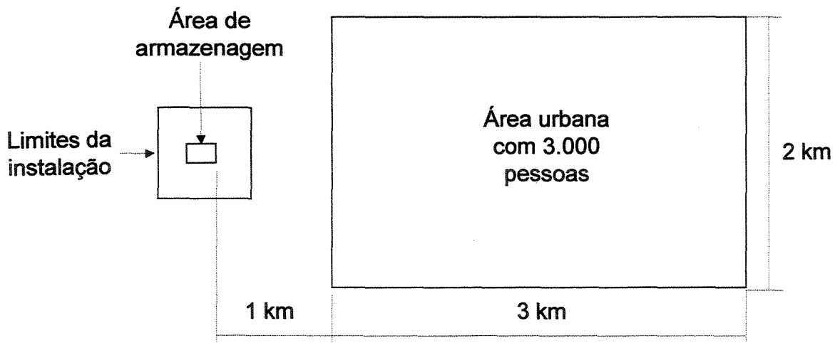
Figura 5.3 - Leiaute da instalação de armazenagem de UO_2 , com enriquecimento de 5 % em U-235.
